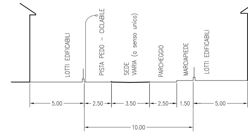
SEZIONE STRADALE C SCALA 1:200
