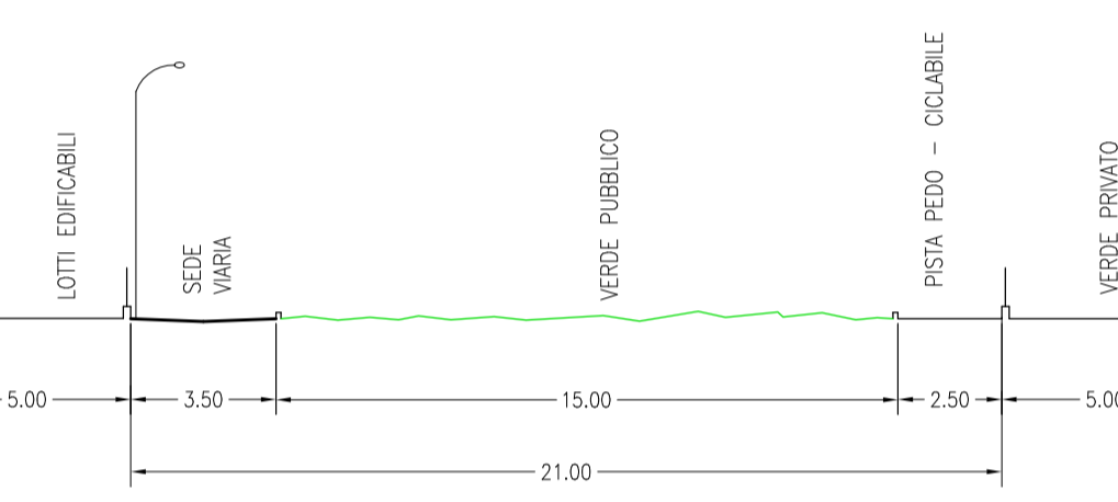
SEZIONE STRADALE F SCALA 1:200
