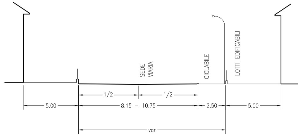
SEZIONE STRADALE E SCALA 1:200
