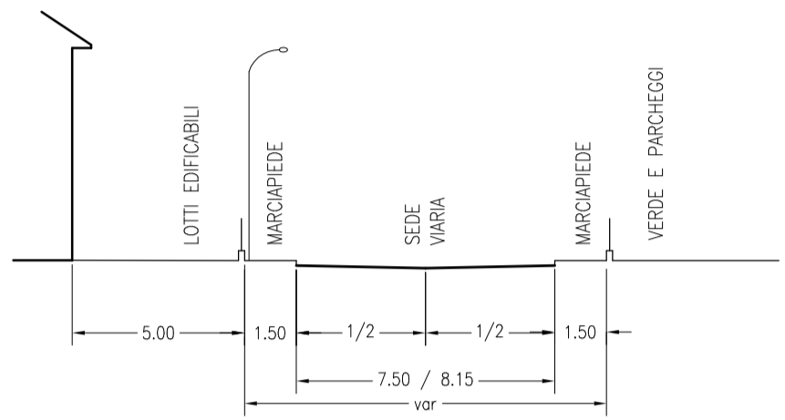
SEZIONE STRADALE B SCALA 1:200
